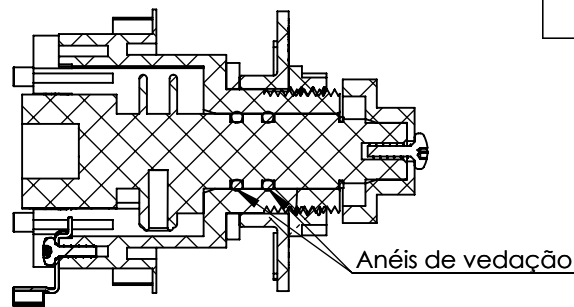
SEÇÃO A-A
