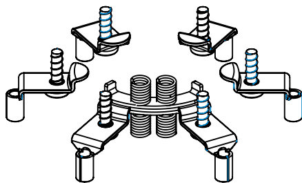
Duplo fechamento dos contatos (sistema deslizante)
